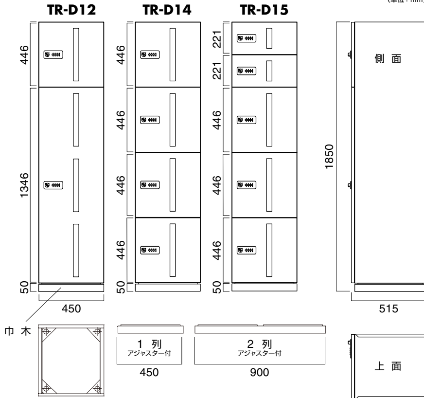
ボックス内部寸法 (単位: mm)
